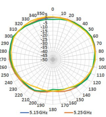
Radio2 5.0 GHz 垂直面
