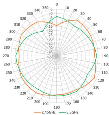
Scanning Radio 水平面
