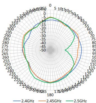
BLE Radio 水平面
